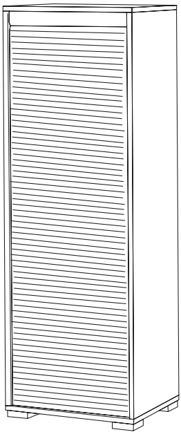
1633/45.949 L 46 - PR 35 - H 141 MULTIUSO SERRANDINA 1 RIPIANO FISSO 2 RIPIANI REGOLABILI COLORI: BIANCO FRASSINO
